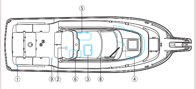
■外観図
